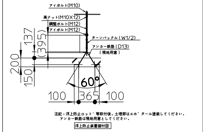
浮上防止金具(オプション例)
