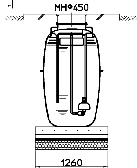
右側面図
