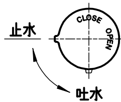
矢視A
