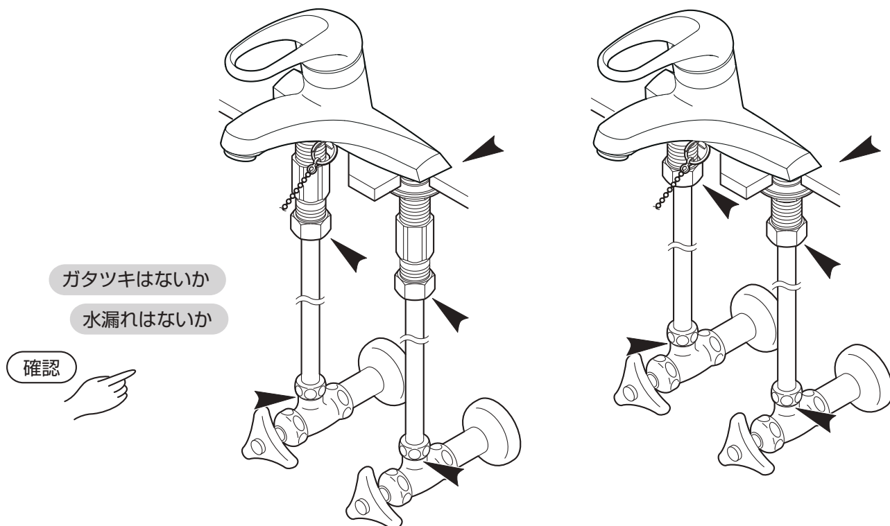
逆止弁あり
