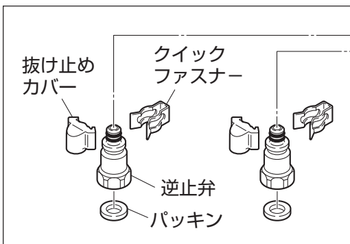
逆止弁 ×2
