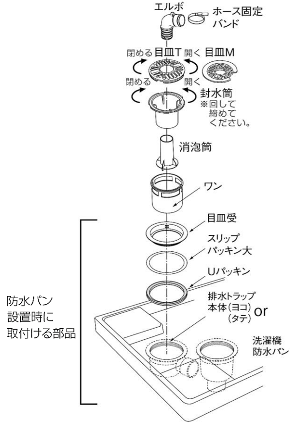
●トラップ組立図 ※図2
