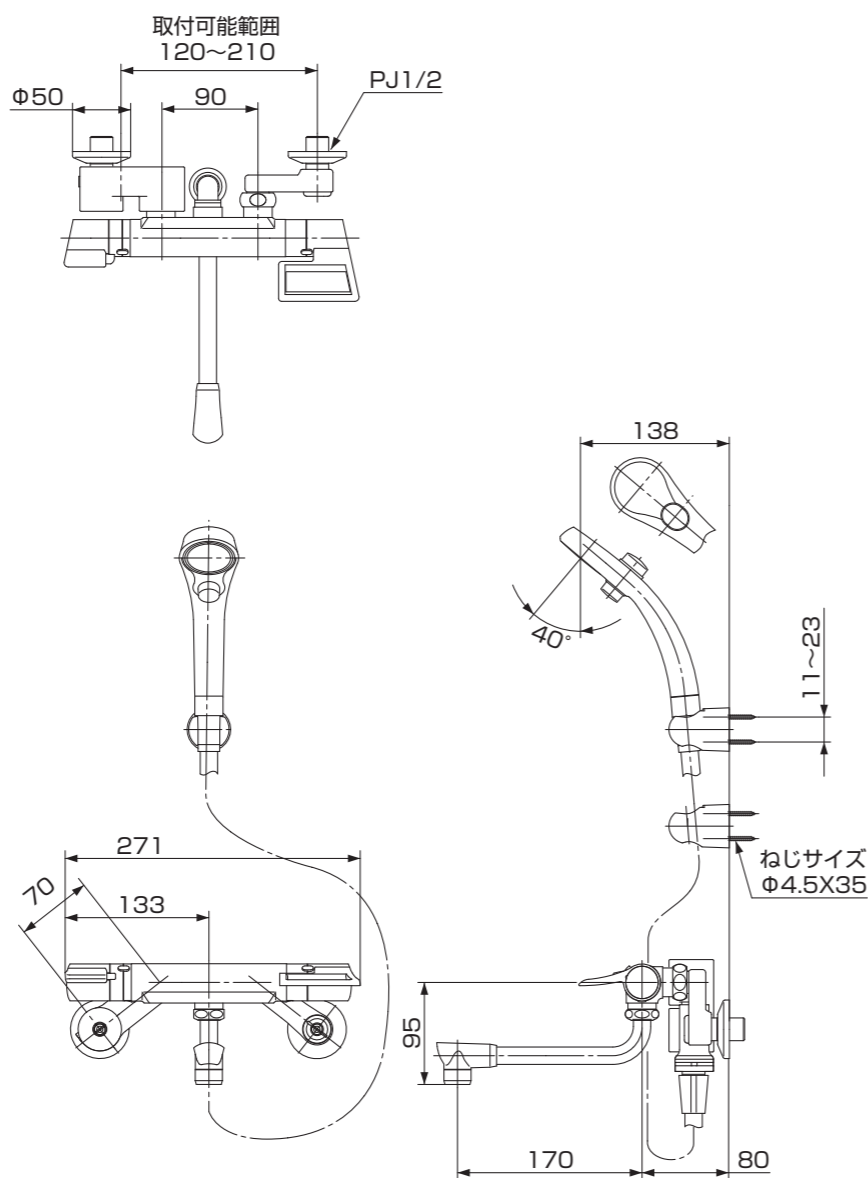
(施工例：SK1813DT2-13)
