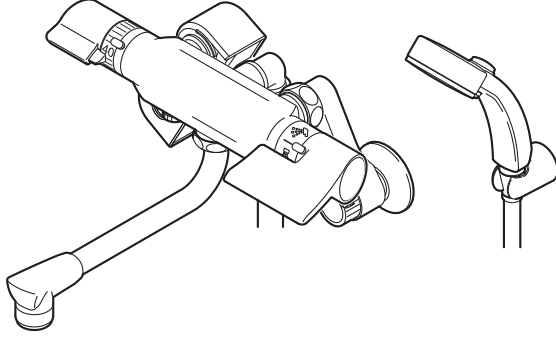
(施工例：SK181ADCT5-13)
