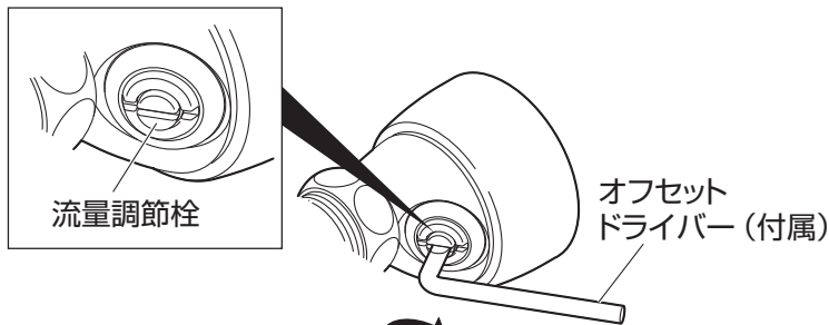
1 流量調節栓
