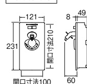
屋内用混合栓
