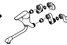
既設偏心管に取付け
