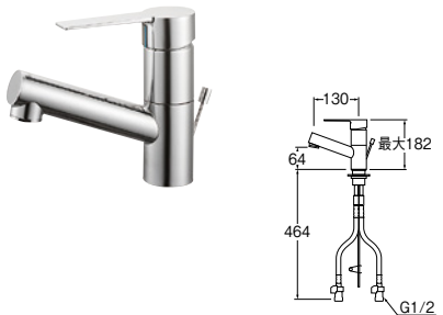
フラット吐水
