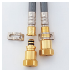
フレキホース クイックファスナー
