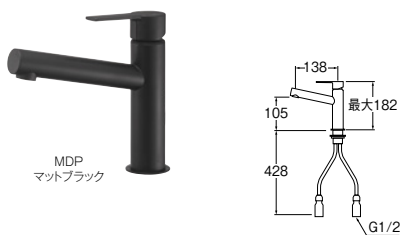
フラット吐水
