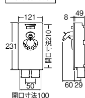
屋内用混合栓
