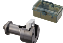
R8310 ¥46,000 1-5 巻ベンリーカンツバ出し機 ・T13・T19巻ベンリーカン兼用 ・呼び13X16、13X16.8、20兼用 ・ケース付
