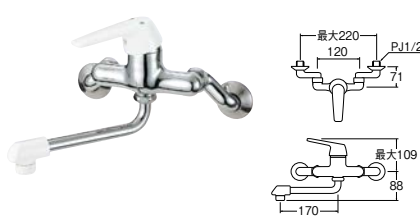
㊦ シングル混合栓
