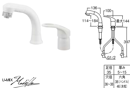
㊦ シングルスプレー混合栓（洗髪用）
