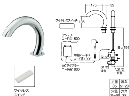
㊦ サーマ混合栓（ワイヤレススイッチ付）
