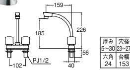
㊤ ツーバルブ台付混合栓 [共用形]
