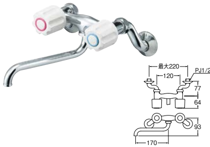
⑨ ツーバルブ混合栓 [共用形]
