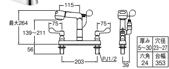
㊤ ツーバルブ台付スプレー混合栓
