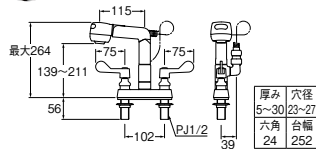
㊤ ツーバルブ台付スプレー混合栓
