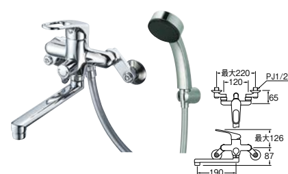
⑬ シングルシャワー混合栓
