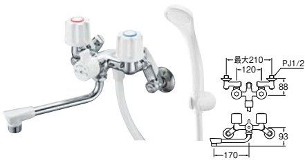
⑨ ツーバルブシャワー混合栓 (一時止水)
