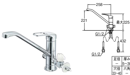
㊦シングルワンホール分岐混合栓
