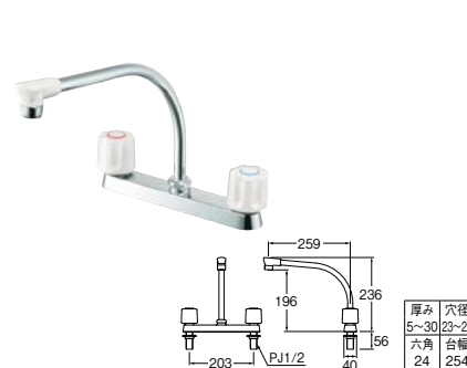
㊦ ツーバルブ台付混合栓 [共用形]
