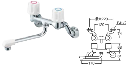
⑨ ツーバルブ混合栓 [共用形]
