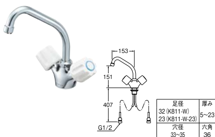
㊦ ツーバルブワンホール混合栓
