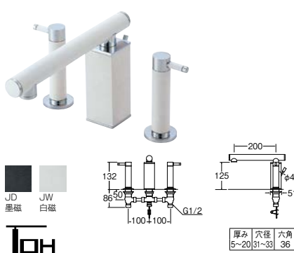
⑨ツーバルブ洗面混合栓
