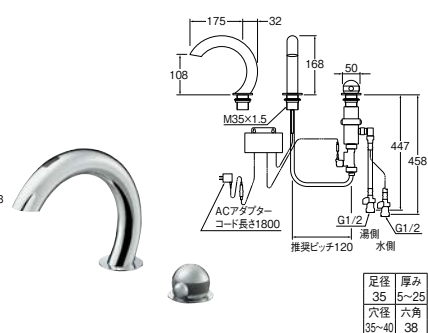
㊦ サーマ付自動洗面混合栓
