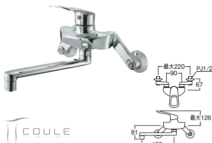
㊦ シングル混合栓
