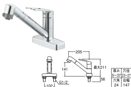
㊦ シングル台付切替シャワー混合栓
