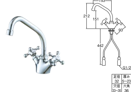
⑨ツーバルブワンホール混合栓
