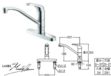
㊦ シングル台付分岐混合栓
