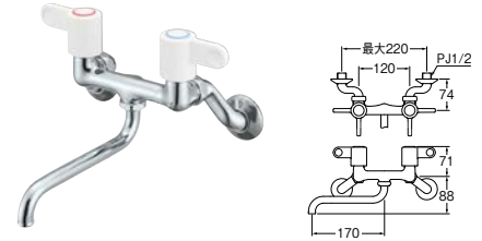
⑨ ツーバルブ混合栓
