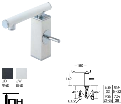
⑨シングルワンホール洗面混合栓
