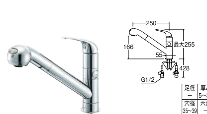
㊦シングルワンホールスプレー分岐混合栓
