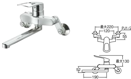
㊦ シングル混合栓
