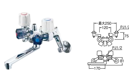
ソーラ4バルブ混合栓
