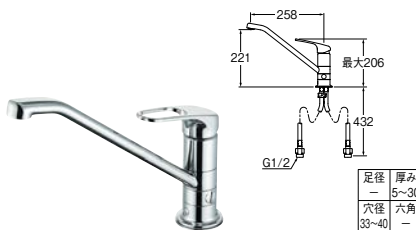
㊦シングルワンホール分岐混合栓
