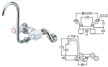
⑨ ツーバルブ混合栓 (折込形) [共用形]
