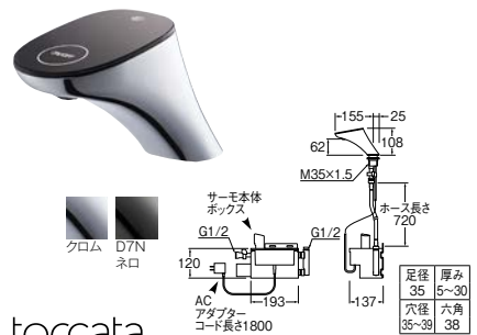
⑨サーモワンホール洗面混合栓 (タッチ式)
