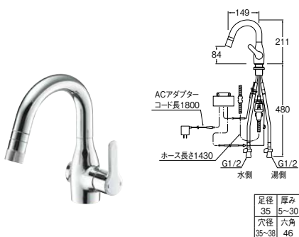
㊦ シングルスプレー混合栓（センサー式）
