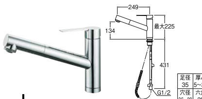
㊦シングルワンホールスプレー混合栓
