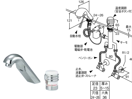
㊦ サーマ付自動混合栓
