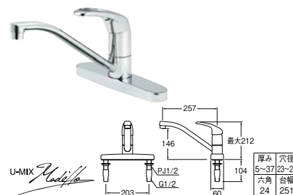
㊦ シングル台付混合栓
