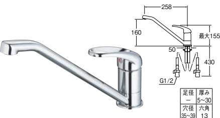
⑨シングルワンホール混合栓
