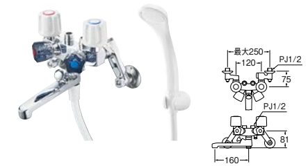
ソーラ4バルブシャワー混合栓
