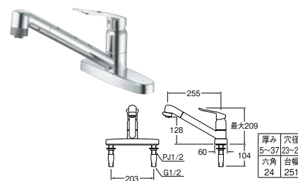
㊦ シングル台付切替シャワー混合栓
