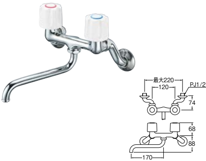
⑨ ツーバルブ混合栓 [共用形]
