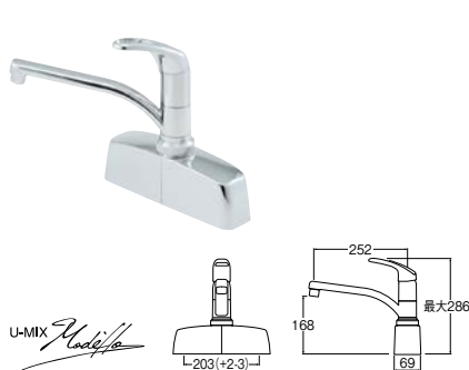
㊦ シングル取替用台付混合栓
