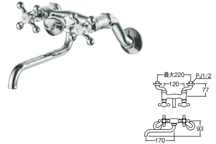
⑨ ツーバルブ混合栓
