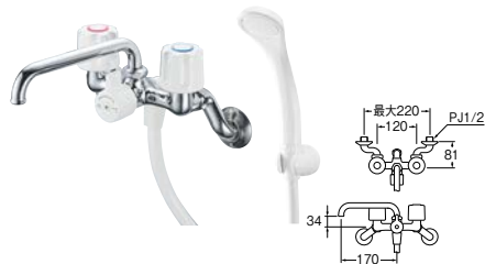
⑨ ツーバルブシャワー混合栓 [共用形]
