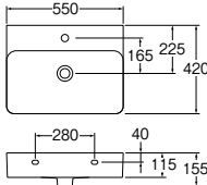
単品図面
