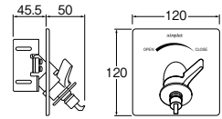
屋内用単水栓
