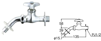
㊤洗濯機用ホーム水栓
