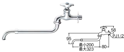
伸縮自在水栓 (固定コマ仕様)
