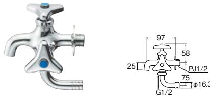
二口横水栓
