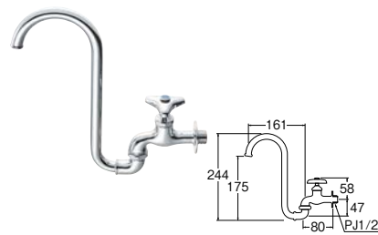
⑨ツル首自在水栓 (固定コマ仕様)
