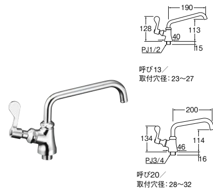
㊤ 厨房用立形上向自在水栓 (左ハンドル) [共用形]
