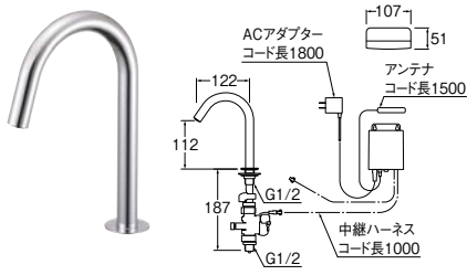
取付穴径: 22~26
