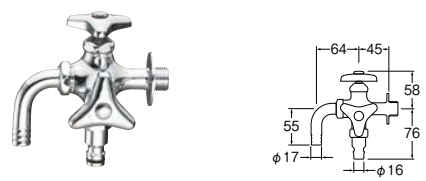
㊦ 散水用二口横水栓
