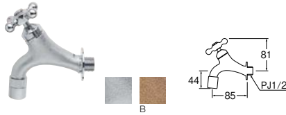
ガーデン水栓 (クロスハンドル)
