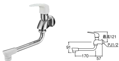
㊦ シングル自在水栓
