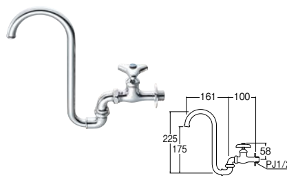
折込形自在水栓 (固定コマ仕様)
