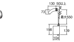
取付穴径: 33~36 厚み 1~15
