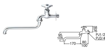
㊦ 自在水栓 (固定コマ仕様)
