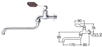
⑨節水レバー自在水栓 (固定コマ仕様)
