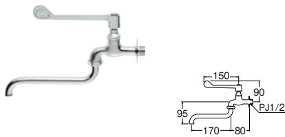
⑨レバー式自在水栓 (吊コマ仕様)
