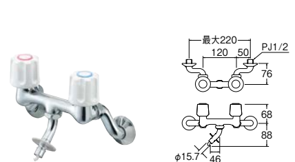
㊤ツーバルブ洗濯機用混合栓
