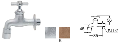
ガーデン水栓 (一文字ハンドル)
