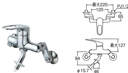
㊤シングル洗濯機用混合栓
