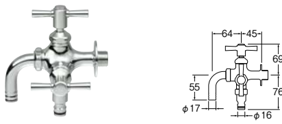
㊦ 散水用二口横水栓
