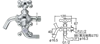
㊦ 万能二口横水栓 (固定コマ仕様)
