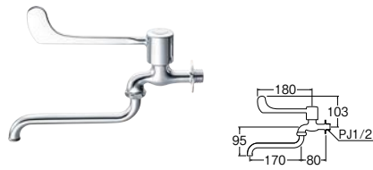
⑨レバー自在水栓 (吊コマ仕様)
