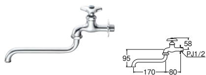
㊦ 自在水栓 (節水固定コマ仕様)
