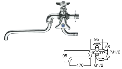
二口自在水栓
