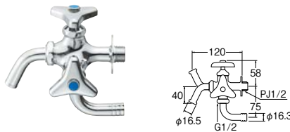
万能二口横水栓
