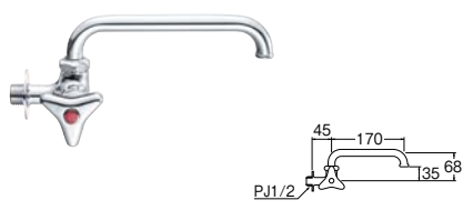
⑨横形自在水栓 (左ハンドル) (固定コマ仕様)
