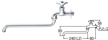
㊦ 自在水栓 (固定コマ仕様)
