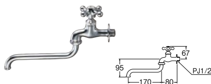
㊦ 自在水栓 (固定コマ仕様)
