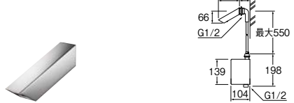
取付穴径: 22~24 厚み 1~25
