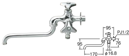
㊦ 散水用二口自在水栓
