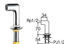
水栓取付脚 L
