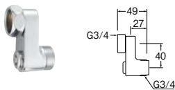
後付け偏心管
