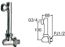
延長偏心管
