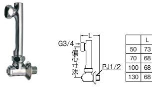
延長偏心管
