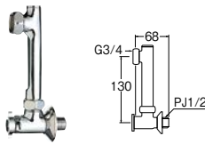
延長偏心管
