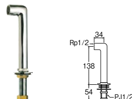
水栓取付脚 LL
