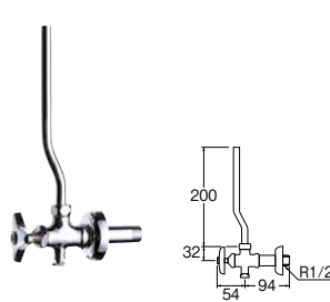
㊦ アンゲル止水栓
