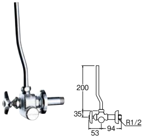
㊦ 逆止付アンゲル止水栓
