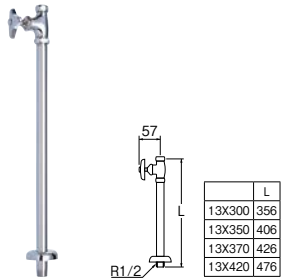
㊦ストレート形止水栓 [共用形]
