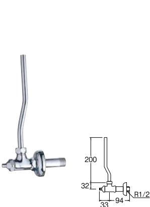
㊦ D式アンゲル止水栓 [共用形]
