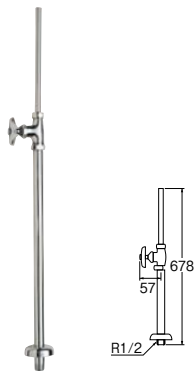
㊦ストレート形止水栓 [共用形]
