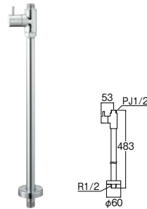
㊦ストレート形止水栓 [共用形] (ヘリューズナシ)
