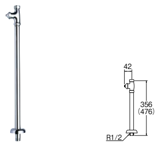
㊦D式ストレート形止水栓 [共用形]
