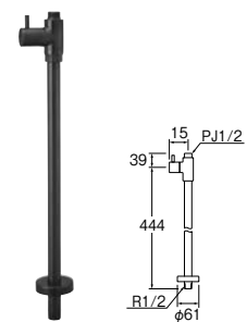
㊦ストレート形止水栓 [共用形]
