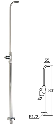
㊦D式L管付ストレート形止水栓 [共用形]
