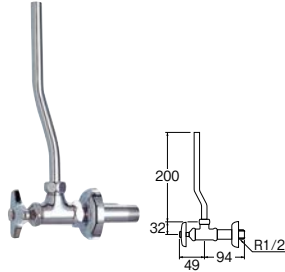
㊦ アンゲル止水栓 [共用形]
