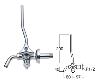
D式アンゲル分岐止水栓(固定コマ仕様)
