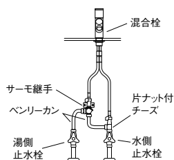
シングルレバー混合栓への配管例
