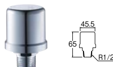
水撃低減器
