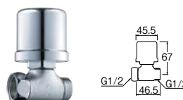
水撃低減器
