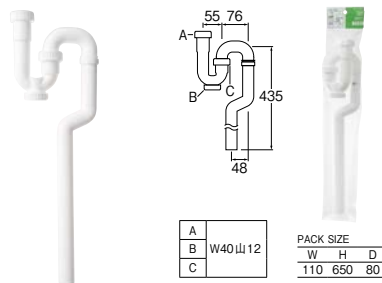
偏心Sトラップ
