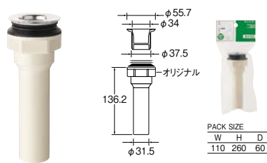
丸鉢排水栓
