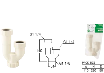
U管
