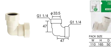
トラップ用エルボ
