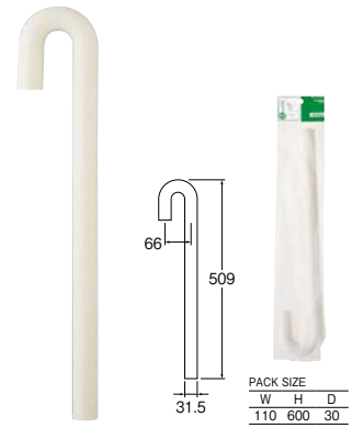
Sパイプ
