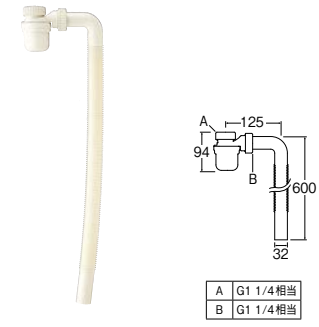
ボトルトラップセット
