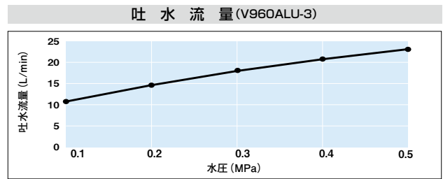
給水圧力/0.1MPa 水温/約20℃ ハンドル全開
