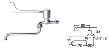
⑭レバー自在水栓 (吊コマ仕様) [共用形]
