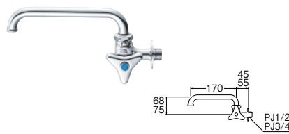
⑱横形自在水栓 (固定コマ仕様) [共用形]
