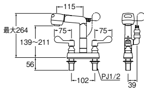
㊦ ツーバルブ台付スプレー混合栓
