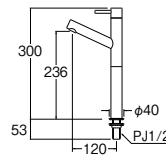
取付穴径: 22~26
