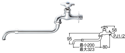
伸縮自在水栓 (固定コマ仕様) [共用形]
