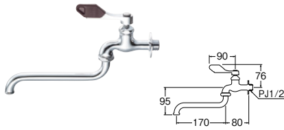
⑬節水レバー自在水栓 (固定コマ仕様) [共用形]
