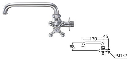
⑰横形自在水栓 (固定コマ仕様) [共用形]
