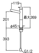
取付穴径: 32~35 取付ロックナット対応: 36
