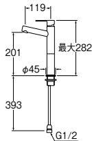
取付穴径: 33~35 取付ロックナット対応: 36
