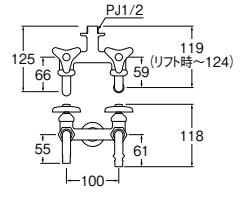
㊦ 散水用二口ホーム水栓 (固定コマ仕様)
