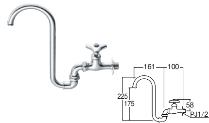
折込形自在水栓 (固定コマ仕様) [共用形]
