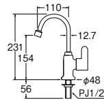
取付穴径: 22~27
