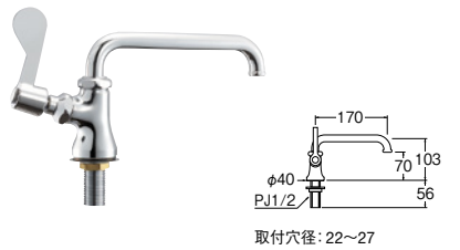
㊦ 厨房用立形自在水栓 (左ハンドル) [共用形]
