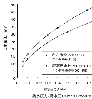
■二条ネジ仕様の吐水量比較データ
