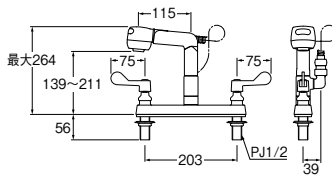
㊦ ツーバルブ台付スプレー混合栓
