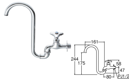
⑯ツル首自在水栓 (固定コマ仕様) [共用形]
