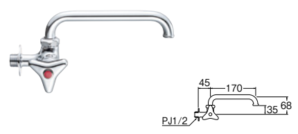
⑲横形自在水栓 (左ハンドル) (固定コマ仕様) [共用形]
