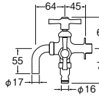
㊦ 散水用二口横水栓 (固定コマ仕様)
