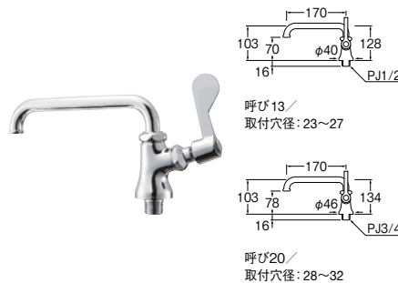
厨房用立形自在水栓 [共用形]
