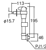
㊦ミニセラ洗濯機用水栓
