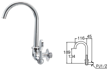
㊦ 厨房用横形ツル首自在水栓 [共用形]
