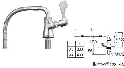
厨房用ベンリー立形自在水栓 [共用形]
