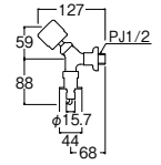
水撃低減洗濯機用送り座水栓(固定コマ仕様)
