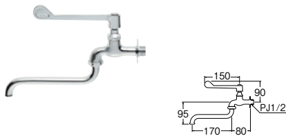
⑮レバー式自在水栓 (吊コマ仕様) [共用形]
