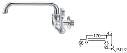
㊦ 厨房用横形自在水栓 [共用形]
