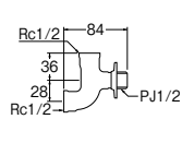
二又ソケット (POS) JB10A-13 ¥5,200 5-50
