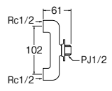
二又ソケット (POS) JB13A-13 ¥5,400 5-50
