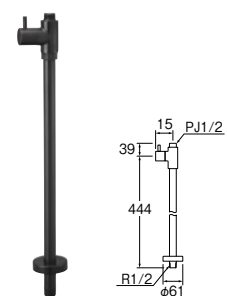
㊸ストレート形止水栓 [共用形]
