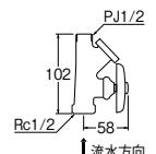
㊦ストレーナ45°化粧バルブ [共用形] V29-1-13 ¥6,200 2-40 ・ストレーナ内蔵 ・#60、線径φ0.18
