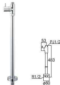
㊸ストレート形止水栓 [共用形] (ヘリューズナシ)
