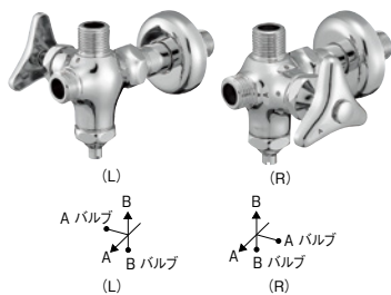
㊸ D式分岐止水栓本体 [共用形]
