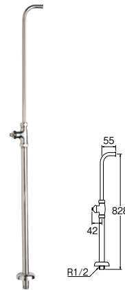
㊸D式L管付ストレート形止水栓 [共用形]
