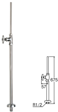
㊸ストレート形止水栓 [共用形]
