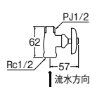
㊦化粧バルブ2型 [共用形] V21A-2-13R ¥4,100 5-40 ・赤ビス仕様
