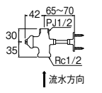
D式止水栓本体 [共用形] V2110D-13X48 ¥6,700 2-40 ・品番の最後は支持棒の長さ ・支持座金、ビス付
