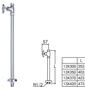
㊸ストレート形止水栓 [共用形]
