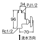
㊦ストレーナ化粧バルブ [共用形] V280A-13 ¥8,300 2-40 ・ストレーナ内蔵 ・#50、線径φ0.18
