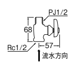
㊦化粧バルブ [共用形] V211-13 ¥3,700 5-40 ・オネジ部分が長く、ブラケットの取り付けに適しています。
