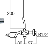
D式アンゲル分岐止水栓 (固定コマ仕様)
