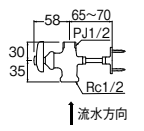
止水栓本体 [共用形] V2110-13X48 ¥6,700 2-60 ・品番の最後は支持棒の長さ ・支持座金、ビス付
