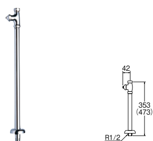
㊸D式ストレート形止水栓 [共用形]
