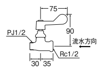
㊦厨房用化粧バルブ [共用形] V2111-13 ¥5,600 1-40 二条ネジ
