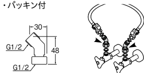
片ナット付45°エルボ (パッケージ品)
